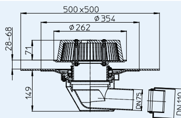
Pralaidumas pagal EN 1253 normatyvus su 3m ilgio vertikaliu nuvedimu Pralaidumas l/s kai nuvedamo vandens lygis nuo 5mm iki 65mm
